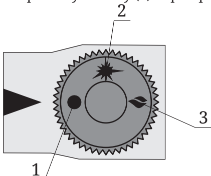
Рисунок 3. Внешний вид ручки управления регулятора подачи газа 820 NOVA
