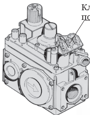
Рисунок 5. Внешний вид энергонезависимого регуля- тора подачи газа 820 NOVA.
