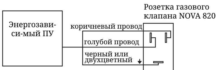
Рисунок 15. Подключение энергозависимой автоматики
